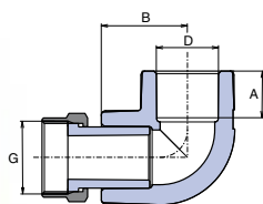
Угольник 90 ° переход с накладной гайкой
